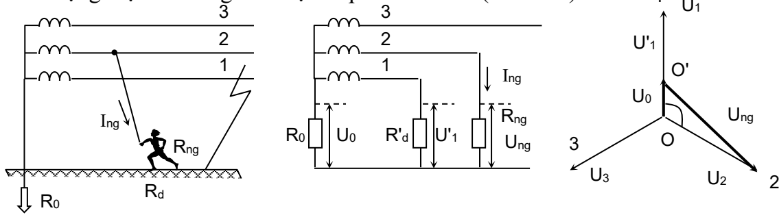
Hình 2-9: Mạng điện ba pha trực tiếp nối đất.
